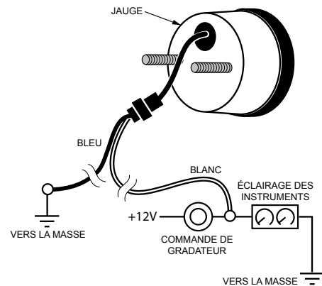
Schéma 2a Pour Les Cdes D'Intensité D'éclairage Sur Positif
